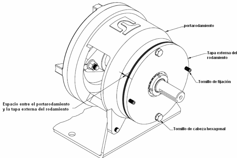
Figura 11 – Ajuste de la tolerancia final
