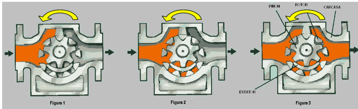
Figura 1 – Principio de bombeo de engranaje interno
