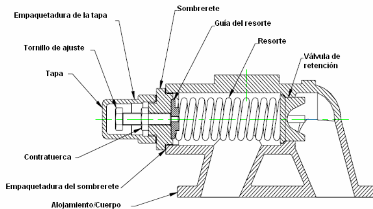
Figura 12 – Válvula de alivio
