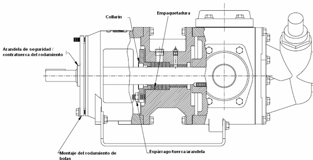
Figura 6 – Bomba con empaquetadura
