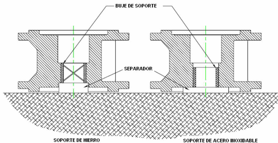
Figura 8 – Bujes de soporte
