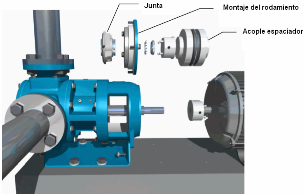
Figura 5 – Cambio de sellos alineados
