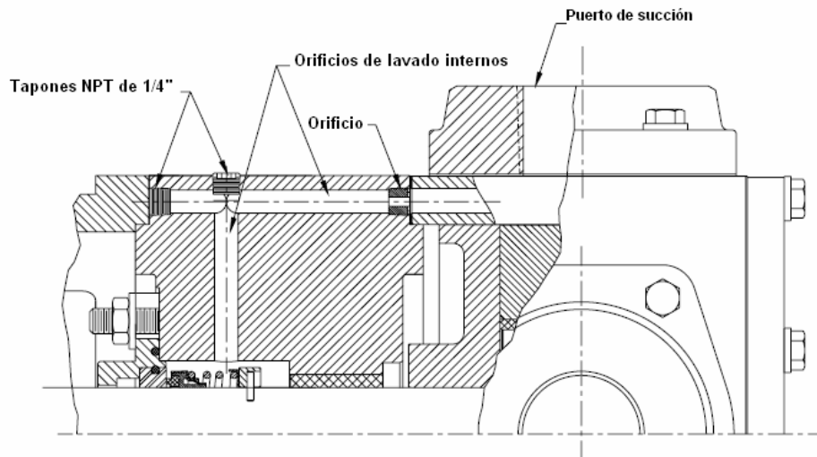
Figura 4 – Ventilación del sello interno
